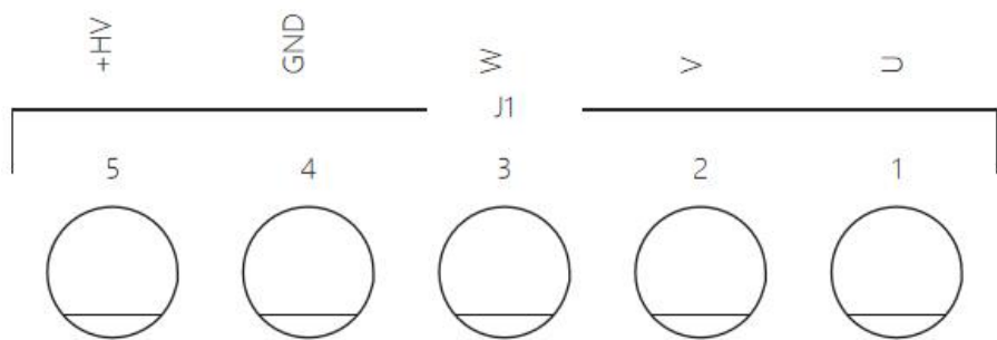
图 2.1 欧规端子
