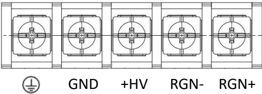
图2.1.2 栅栏端子插座
