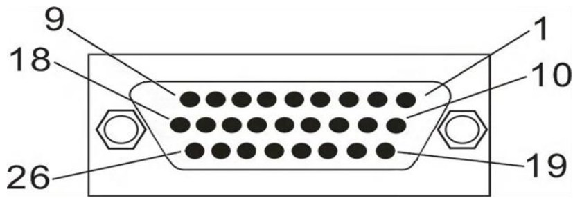
图 3.3 三排 DB26 母座
