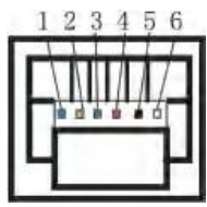
图 3.4 RJ11 6 针水晶头座
