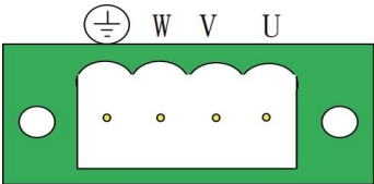
图2.2.1 欧规端子插座
