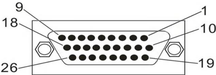
图 2.5 三排DB26母座
