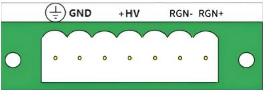
图2.1.1 欧规端子插座
