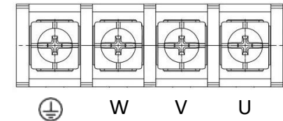
图2.2.2 栅栏端子插座
