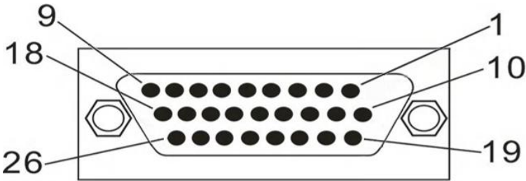
图 2.5 三排DB26母座
