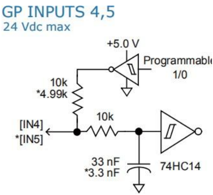
图3.4.2 IN4- IN5硬件输入电路
