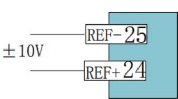
图3.3.2 外部电源模拟量输入接线
