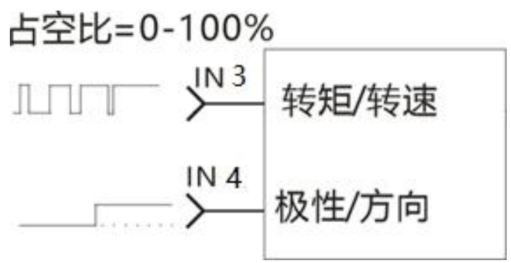
图 3.5 100%占空比+方向控制
