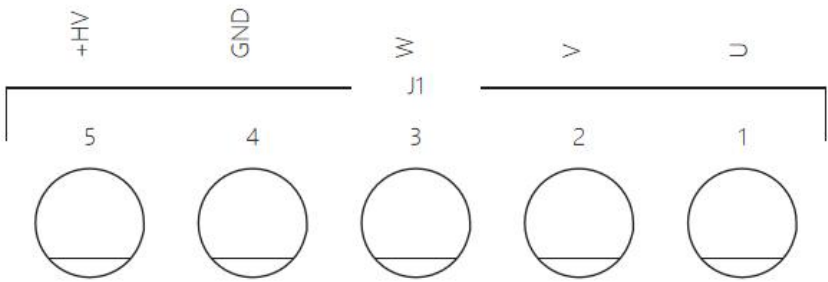
图 2.1.2 J1 端口
