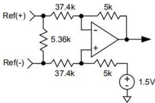
图 3.3.1 模拟量硬件输入电路
