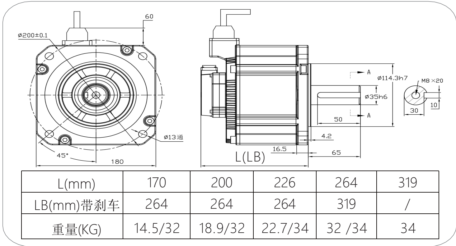
外形尺寸图
