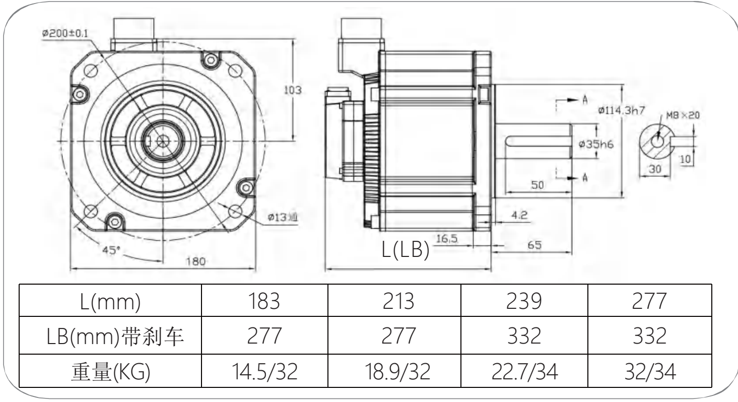
外形尺寸图
