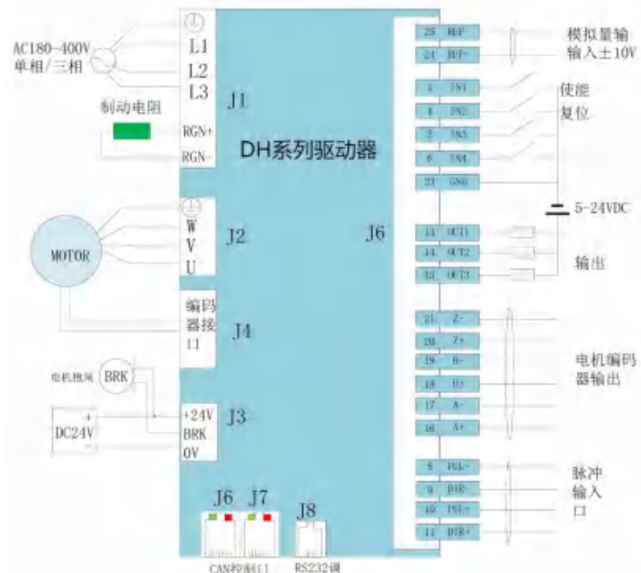
DH380V接线图
