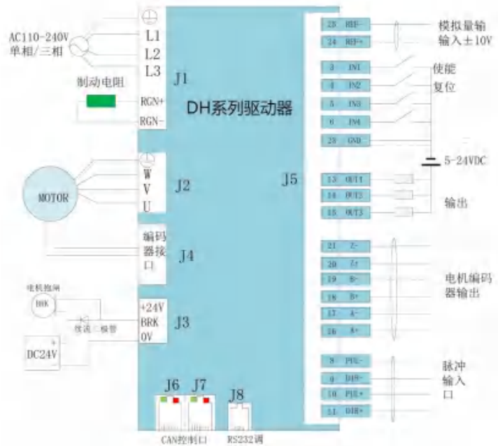
DH220V接线图
